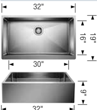
QUATRUS® R15 U 1 MEDIUM APRON
