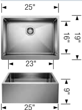
QUATRUS® R15 U 1 MEDIUM APRON
