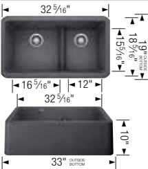
IKON® 33
