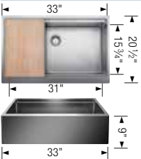
QUATRUS® R15 U 2 APRON
