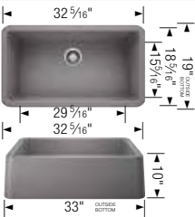
IKON® 30
