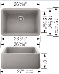
IKON® 27
